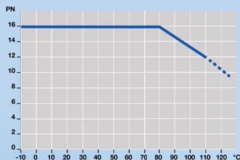
Courbe de pression de service en fonction de la température
